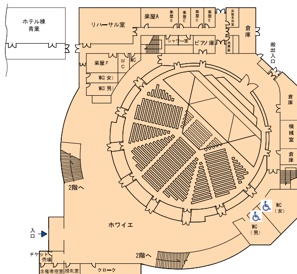
サンプラザホール1階平面図
